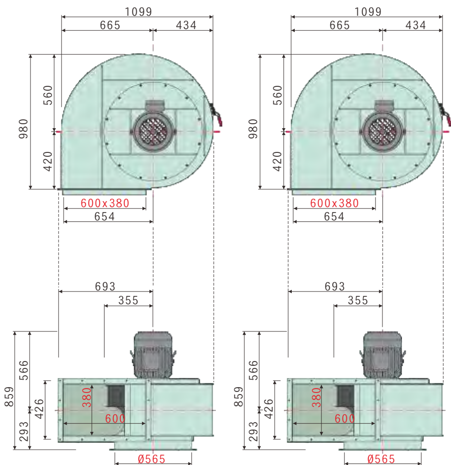
尺寸(毫米) DIMENSIONS(MM) TBNPS-7546
