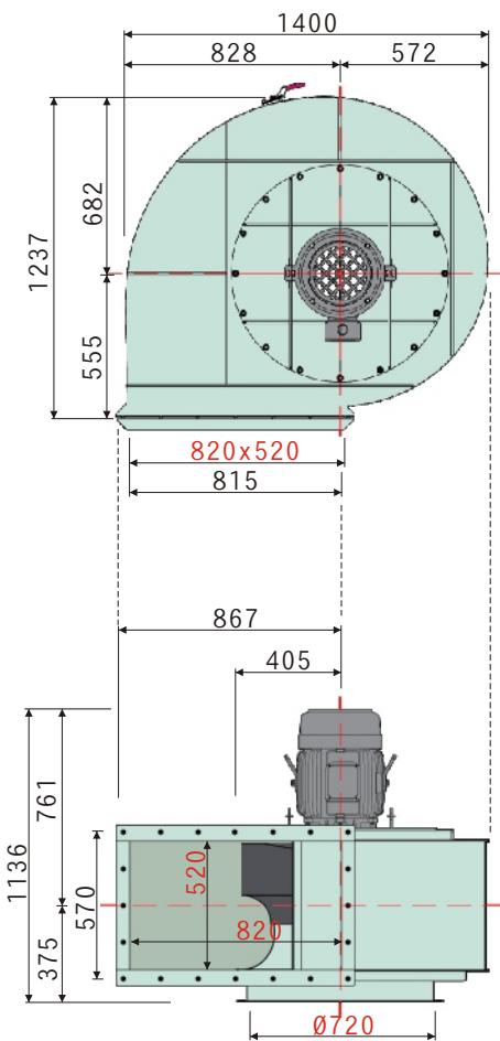
尺寸(毫米) DIMENSIONS(MM) TBNPS-15045
